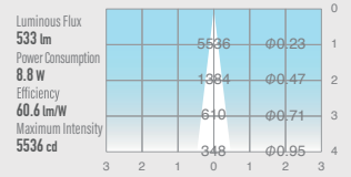
UDL-S75NFGL-40
