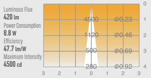
UDL-S75NFGL-27
