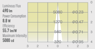
UDL-S75NFGL-30
