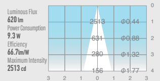
UDL-S75WFGL-40
