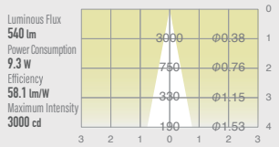
UDL-S75MFGL-30
