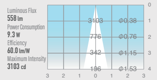
UDL-S75MFGL-40
