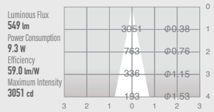
UDL-S75MFGL-35
