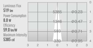
UDL-S75NFGL-35
