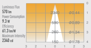
UDL-S75WFGL-27
